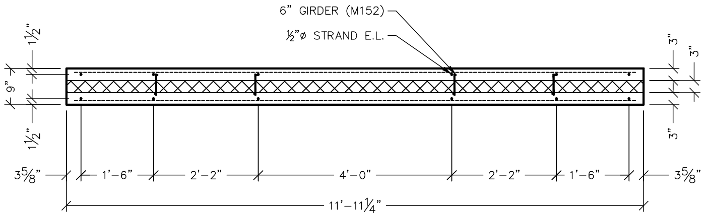
TYP. PANEL & 8' DOCK DOOR SECTION
